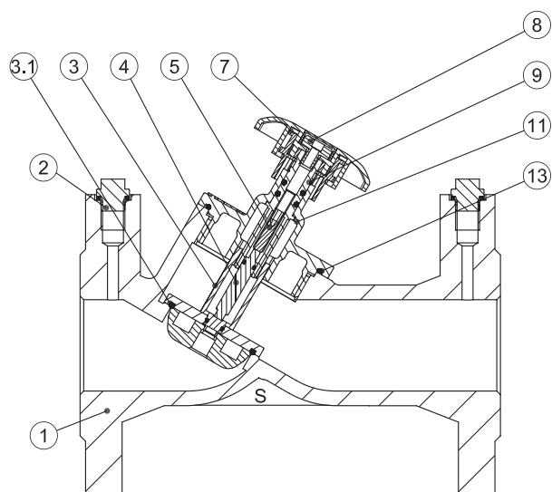
MSV-F2, D_y 50 мм
