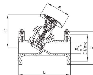
MSV-F2, D_y = 65 мм
