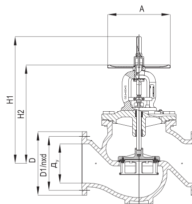
MSV-F2, D_y = 200-300 мм
