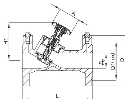
MSV-F2, D_y = 50 мм
