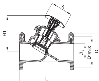
MSV-F2, D_y = 80-150 мм
