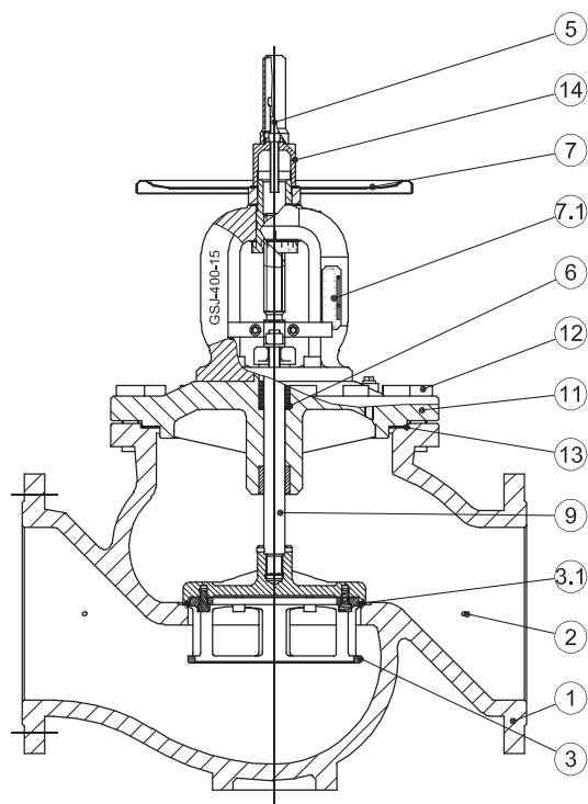
MSV-F2, D_y 200–300 мм
