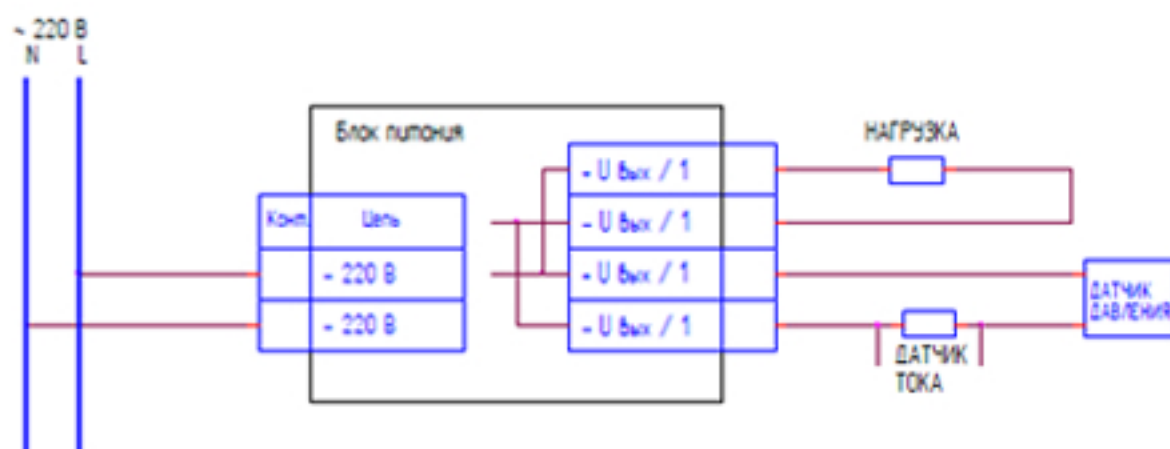
Рисунок Б.1 – Схема включения одноканальных блоков питания в корпусе D3
