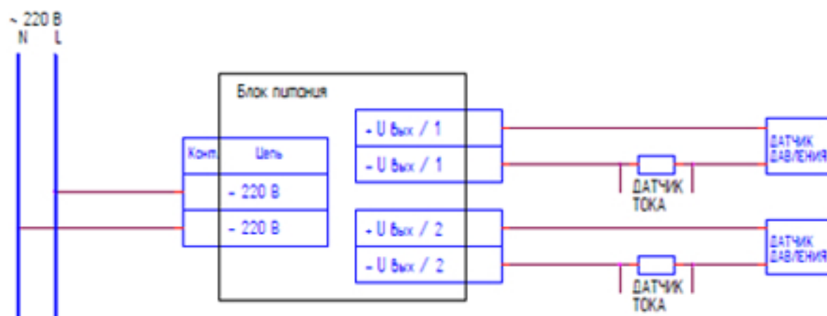
Рисунок Б.4 – Схема включения двухканальных блоков питания
