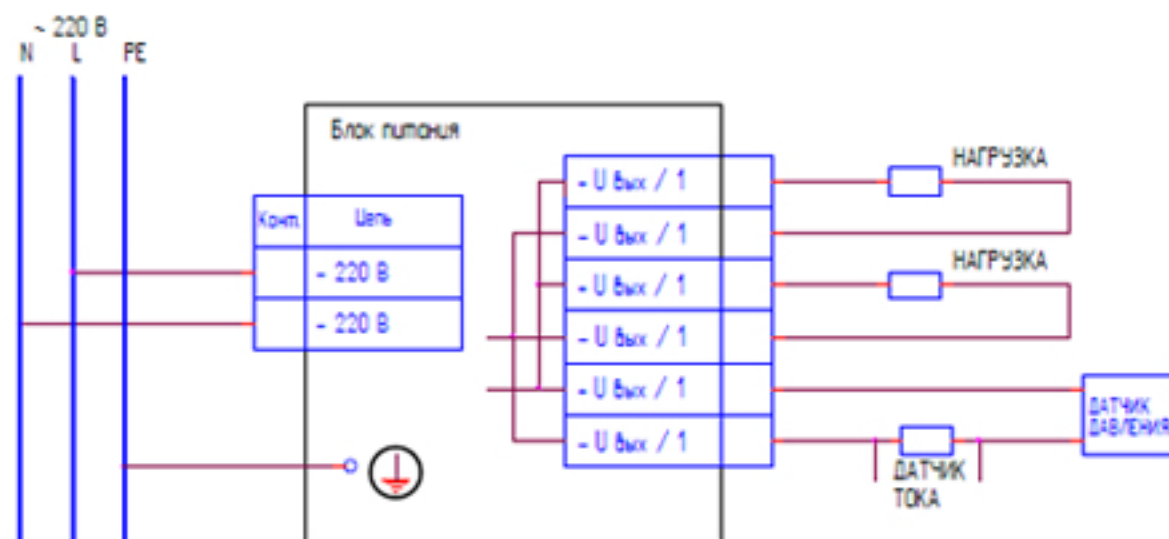
Рисунок Б.3 – Схема включения одноканальных блоков питания в корпусе М
