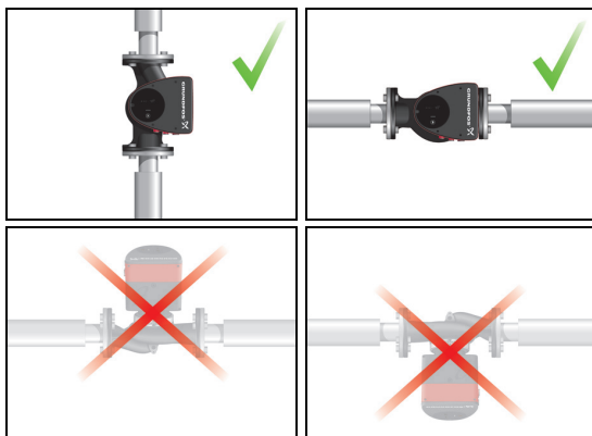
Рис. 16 Варианты монтажа
