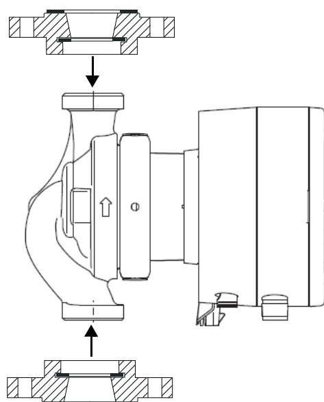
Рис. 29 Пример фланцево-резьбовых переходников
