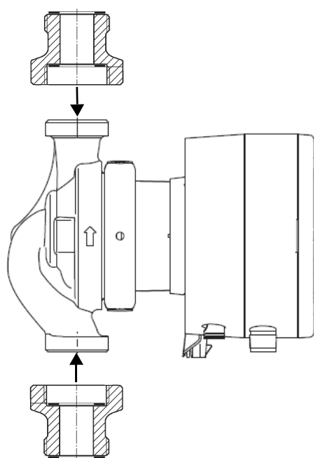
Рис. 27 Пример резьбовых переходников
