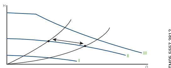
Рис. 9 Три настройки для кривых при фиксированной частоте вращения
