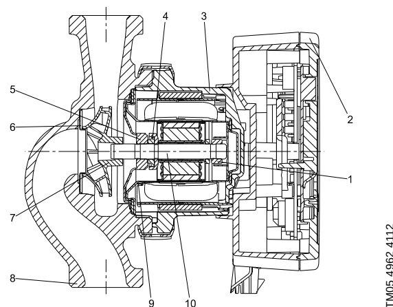
Рис. 15 Модификация с резьбовыми соединениями и корпусом ротора из нержавеющей стали
