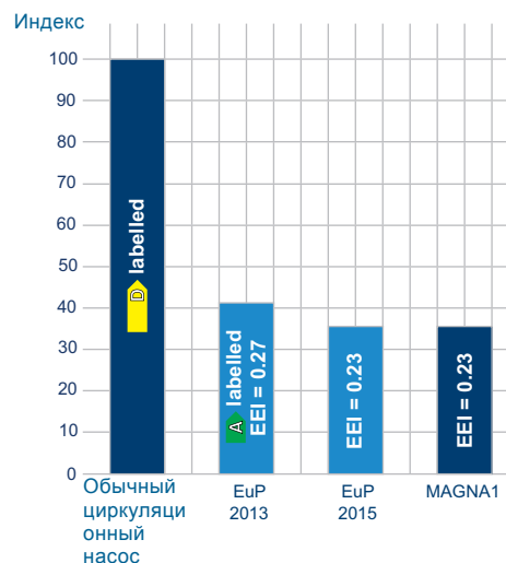
Рис. 22 Индекс энергопотребления
