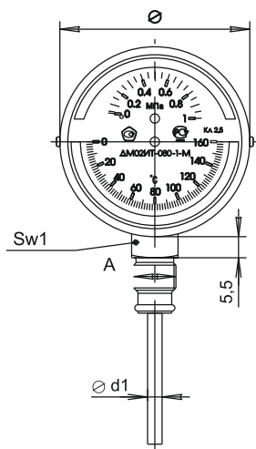
Радиальное исполнение
