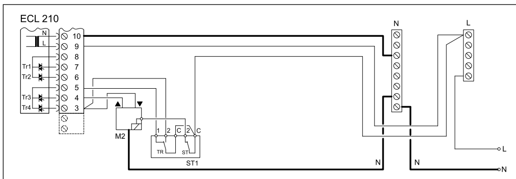
Контур системы ГВС
